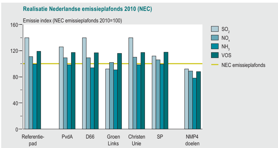
Figuur 4.1 Mate van realisatie van NEC-emissieplafonds en NMP4-doelen 2010, bij uitvoering partijvoornemens van PvdA, D66, GroenLinks, ChristenUnie en SP.
